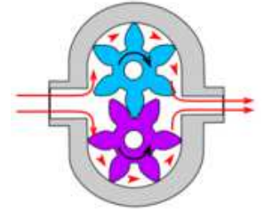
外接歯車ポンプ (油圧機械など)
